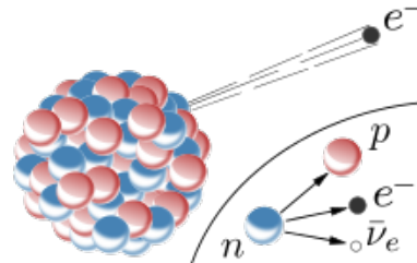
התפרקות רדיואקטיבית ופליטת פרוטון חלקיק בטא (אלקטרון) וקרינת גמא
