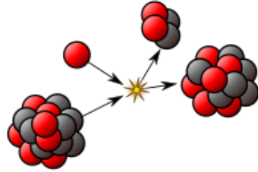
פיצוח גרעין ע"י ניוטרון
